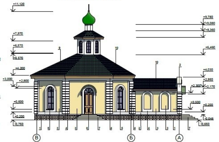
Боковой фасад М 1:100
