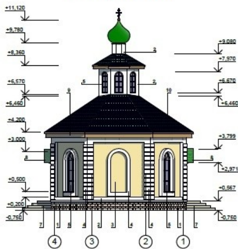
Задний фасад М 1:100
